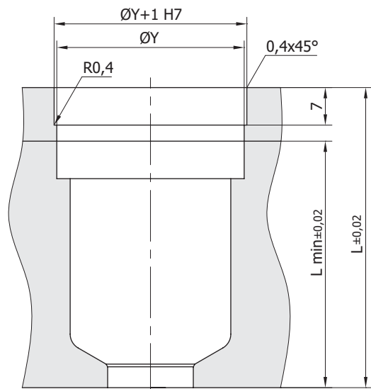
Zabudowa dyszy w tulejach TZO + TZG
